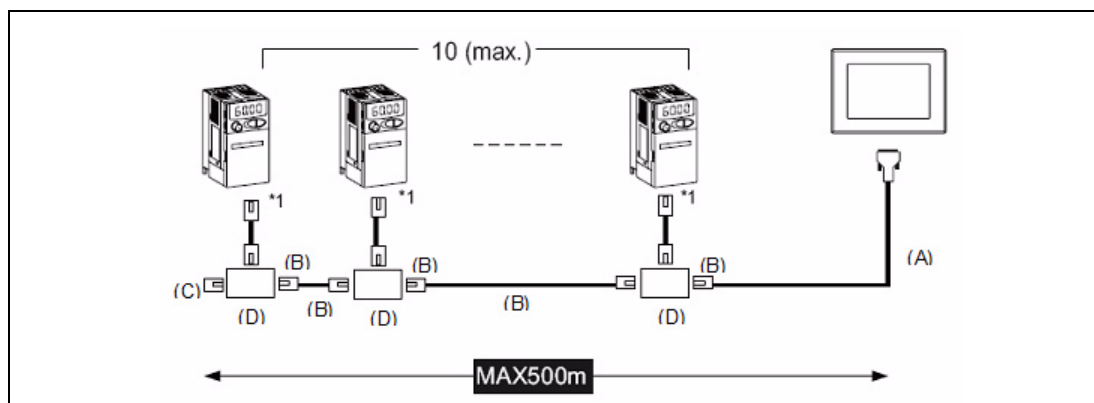
Рис. 2: Многоточечное соединение
