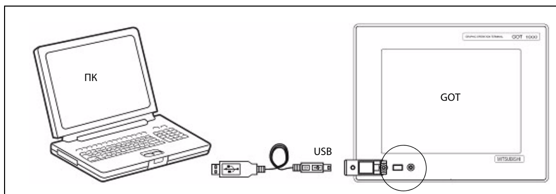
Рис. 3: Схема подключения
