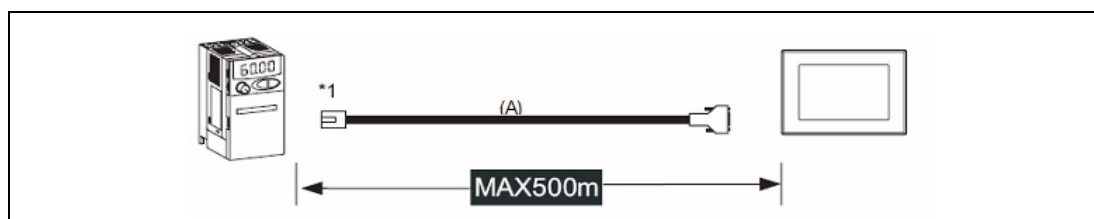
Рис. 1: Соединение с одним преобразователем частоты
